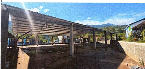
Foto 4: Cubierta de lámina finalizada
